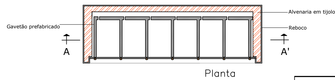
Esquema Montagem Pré - Fabricados
